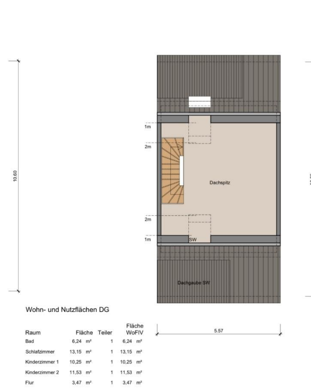
Grundriss Dachgeschoss
